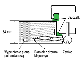
PROFIL SKRZYDŁA PREMIUM
