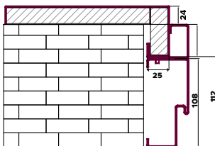
Bande avec cadre réglable IRON
