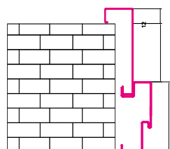
Bande avec cadre interne IRON
