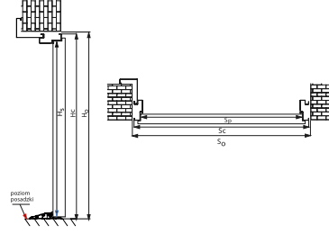
Façon de prise des dimensions de portes IRON avec cadre interne avec portail
