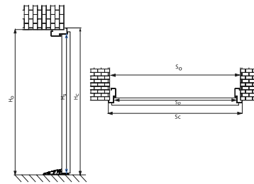
Façon de prise des dimensions de portes IRON avec cadre interne avec portail
