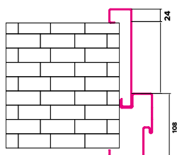
Bande avec cadre réglable IRON
