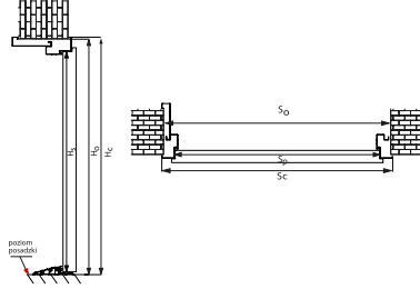
Façon de prise des dimensions de portes IRON avec cadre réglable
