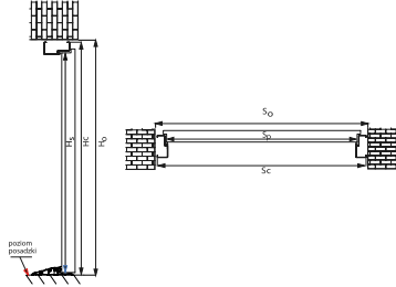
Façon de prise des dimensions de portes IRON avec cadre réglable
