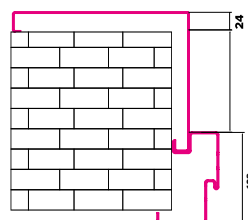
Portail avec cadre réglable IRON
