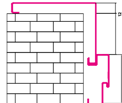
Портал с внутренней коробкой IRON
