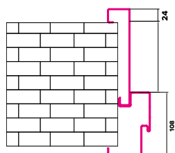
Наличник с регулируемой коробкой IRON
