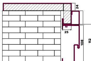
Наличник с регулируемой коробкой IRON
