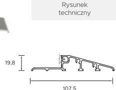
Próg aluminiowy z uszczelką Premium, Normal, Protect, Iron do ościeżnicy "9" (kątovej), "11" (wewnętrznej)
