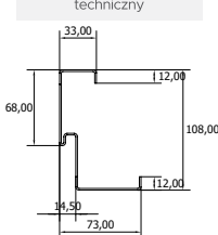
Rysunek techniczny
