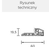
Próg PVC z uszczelką Premium Termo
