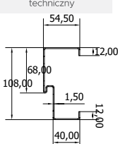
Rysunek techniczny
