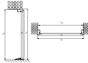
Размеры двери IRON с коробкой под портал
