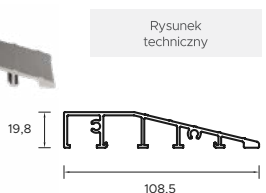
Próg aluminiowy Optimum,
