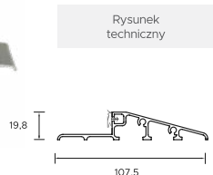
Próg aluminiowy z uszczelką Premium, Normal, Protect, Iron do ościeżnicy "9" (kątovej), "11" (wewnętrznej)
