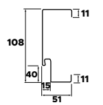
Rysunek techniczny
