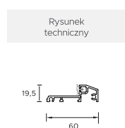
Próg Alu z uszczelką Premium
