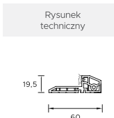
Próg PVC z uszczelką Premium Termo
