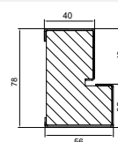
Rysunek techniczny
