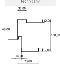
Rysunek techniczny
