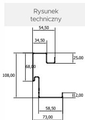
Ciepły próg PVC/ALU z przegrodą termiczną Prestige, Optimum, Premium Plus
