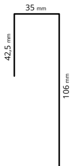
przekrój
