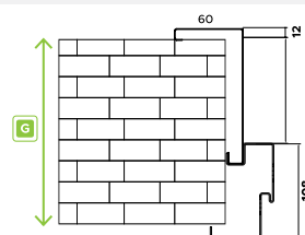
Rysunek techniczny
