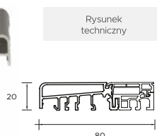
Ciepły próg PVC/ALU z przegrodą termiczną Prestige, Optimum, Premium Plus
