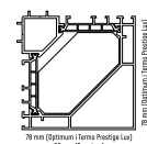
Rysunek techniczny
