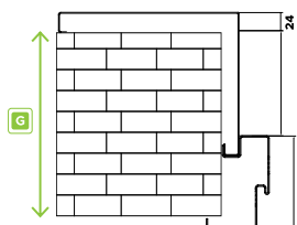
Rysunek techniczny
