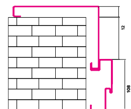
Rahmen mit innerem Türrahmen IRON
