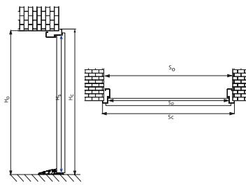
Dimensionierung der IRON-Tür mit Innenzarge für Portal.
