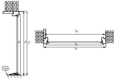
Dimensionierung der IRON-Tür mit verstellbarer Zarge.
