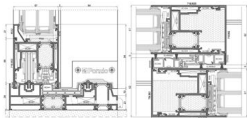
Przekrój okna podnosząco-przesuwne Procural SL1600TT HI
