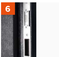
6 Zaczep główny z regulacją języka.
