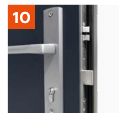
10 Zasuwnica z zam- kiem głównym i wkładką (system jednego klucza).
