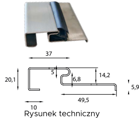
Rysunek techniczny
