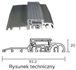
Rysunek techniczny
