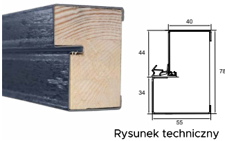
Rysunek techniczny
