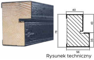
Ościeżnica Stalowo- drewniana Basic 3.0
