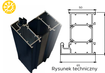
Rysunek techniczny
