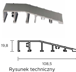
Rysunek techniczny
