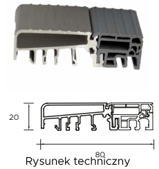
Rysunek techniczny
