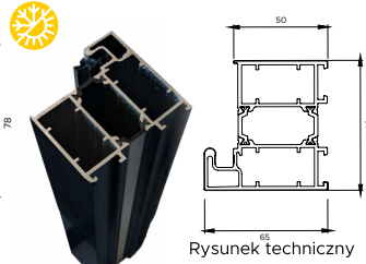
Ościeżnica symetryczna Prima
