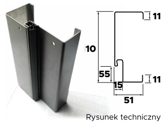
Rysunek techniczny
