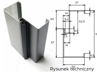
Przekrój łącznika kątowne- go Termo 90°
