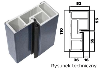
Ościeżnica symetryczna Optimum
