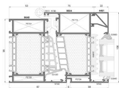
Przekrój okno Procural PE96
