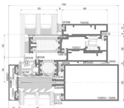
Przekrój Procural PF152HI
