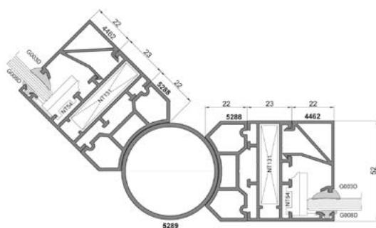
Przekrój ścianki Procural PE50
