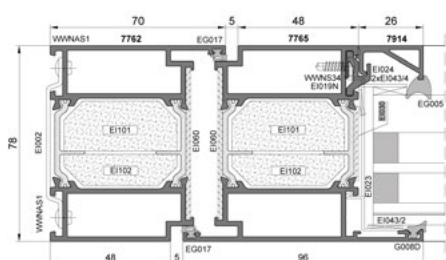
Przekrój PE78EI DESIGN LINE kl. EI30
